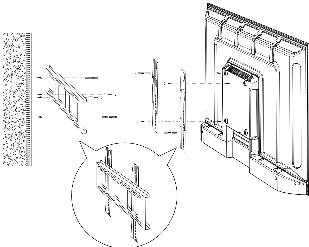
Рисунок 12 – Настенный монтаж телевизора
