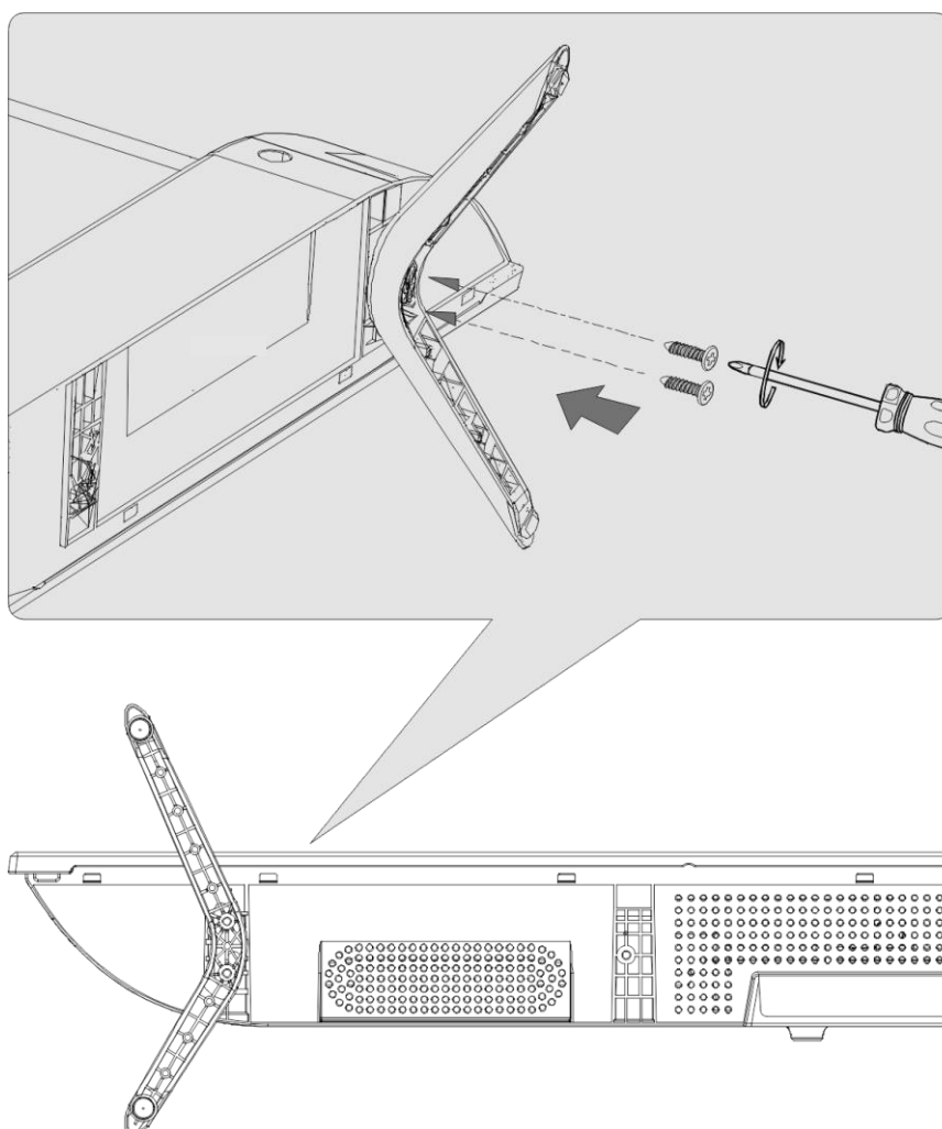
Рисунок 8 – Закрепление двух ножек
